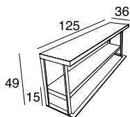
consolle bassa
