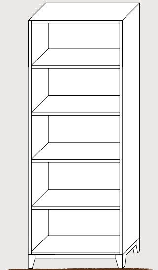
LC012N cm. 70 x 40 x 185 h.
