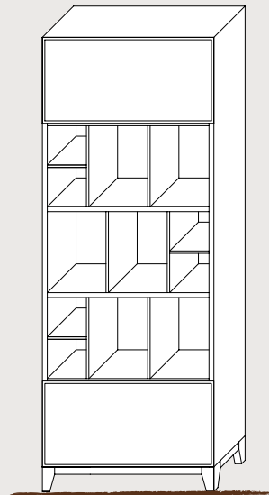
LC052N con 2 ante / with 2 doors cm. 70 x 40 x 185 h.
